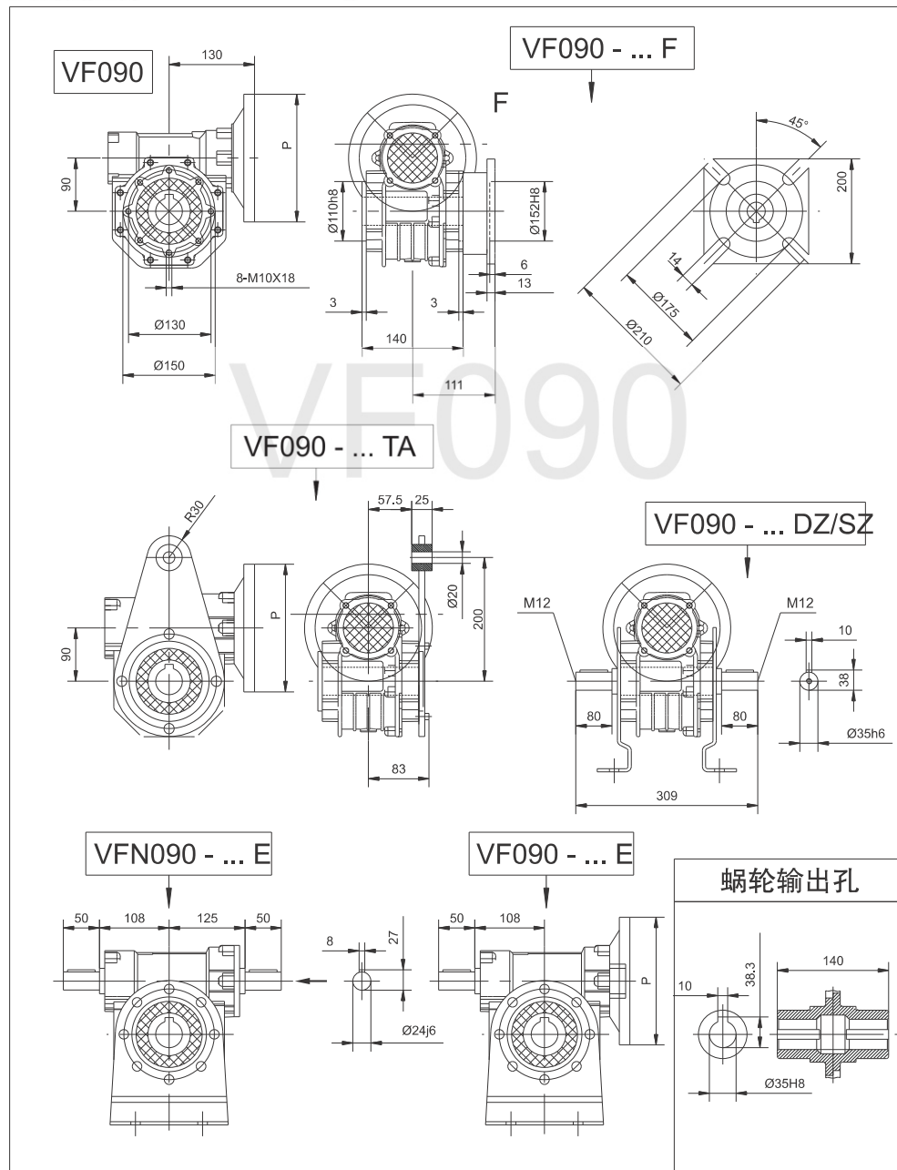
VF090 安装尺寸 P 尺寸见第36页
