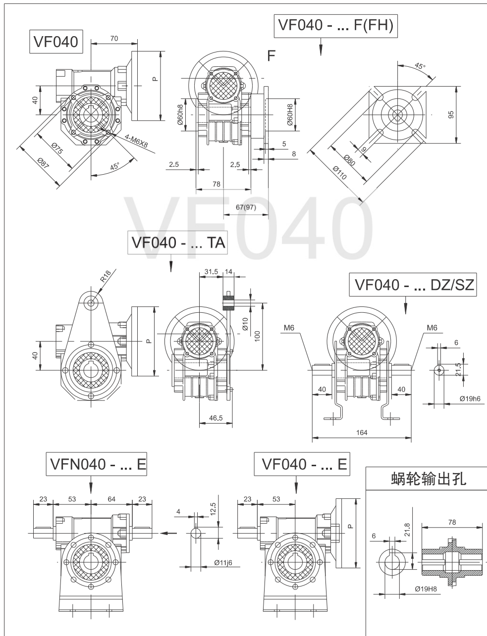
VF040 安装尺寸 P 尺寸见第36页
