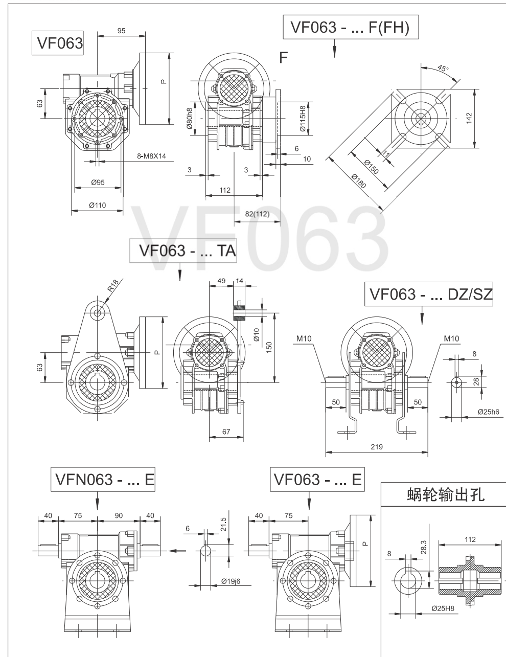
VF063 安装尺寸 P 尺寸见第36页
