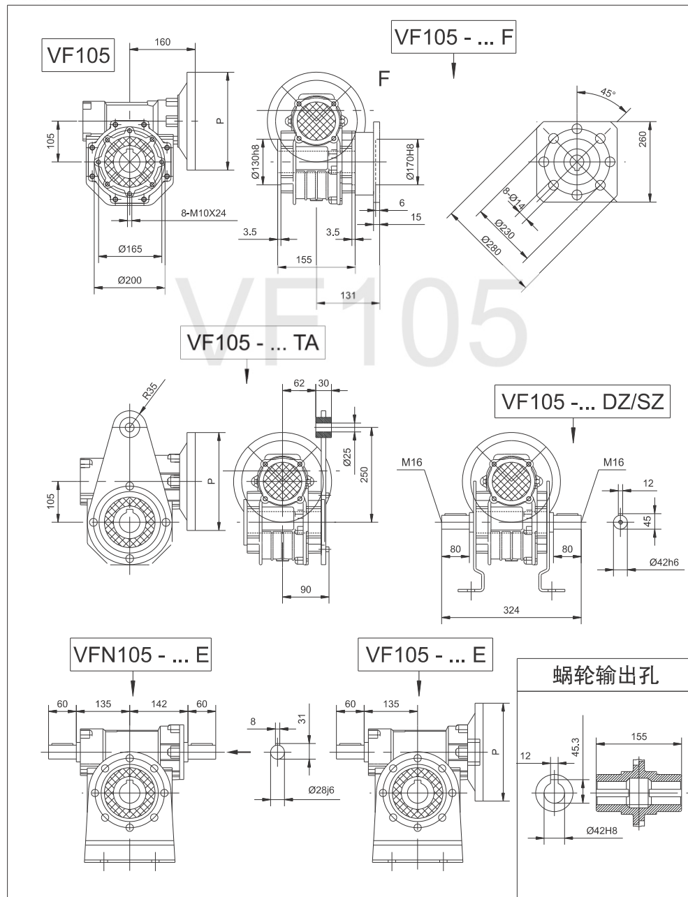
VF105 安装尺寸 P 尺寸见第36页
