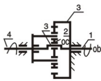
图1 传动原理 Siagram 1 Driving Principe
